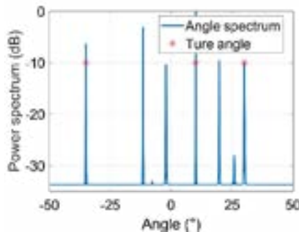
Fig. 6.21 Angle spectrum.
