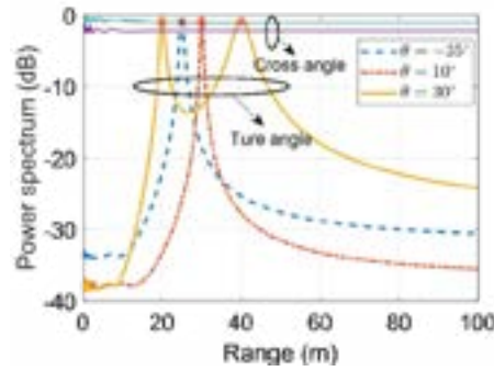
Fig. 6.22 Range spectrum.
